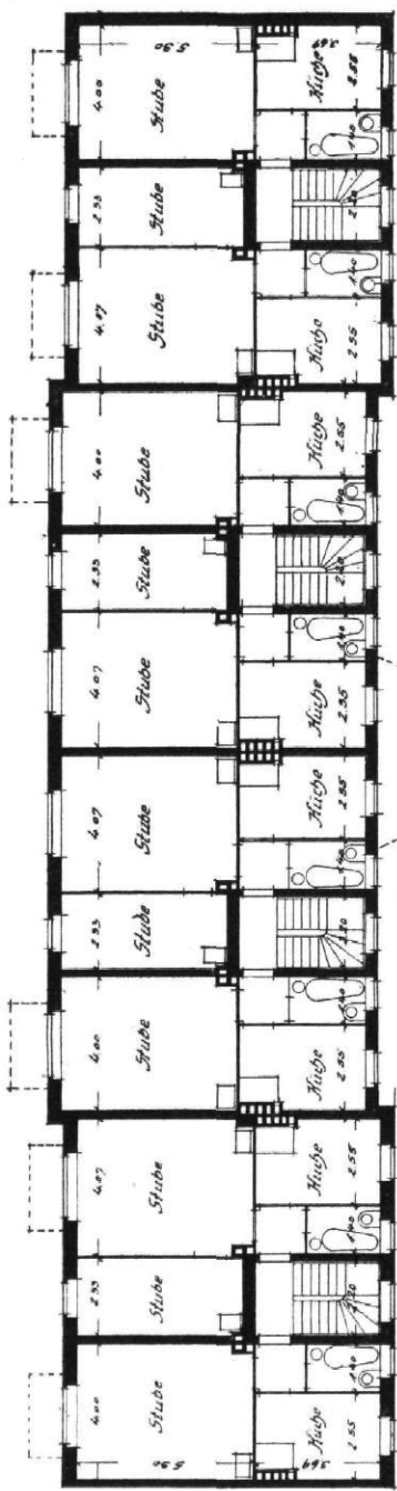
ERDGESCHOSS U. 1. OBERGESCHOSS
