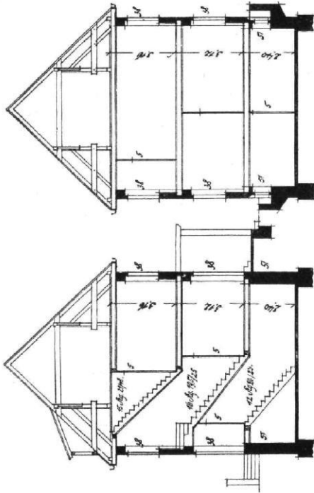
SCHNITTE
