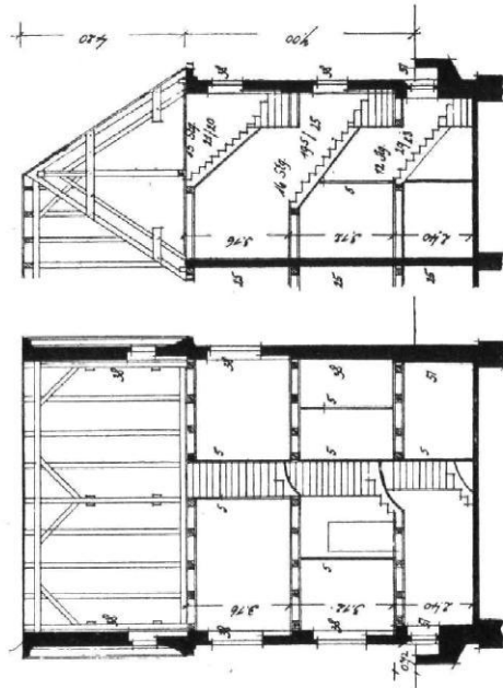
SCHNITTE
