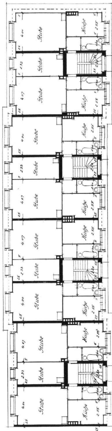
2. OBERGESCHOSS
