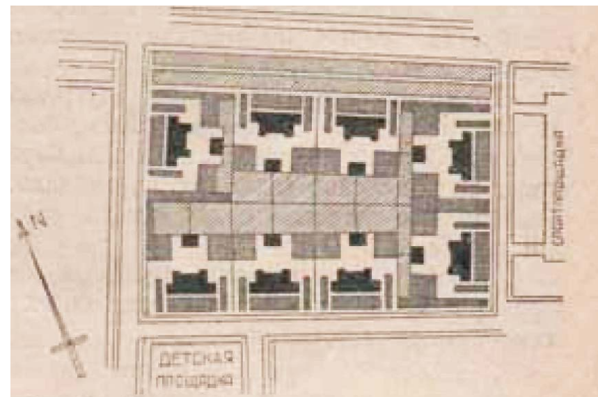
Застройка квартала парными домами
