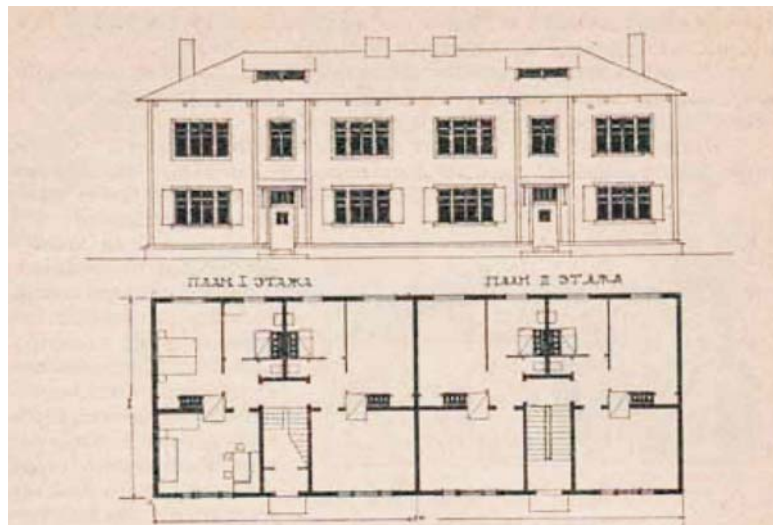
Проект восьмиквартирного дома на Дедовской фабрике Красно-Пресненского треста, тип А
