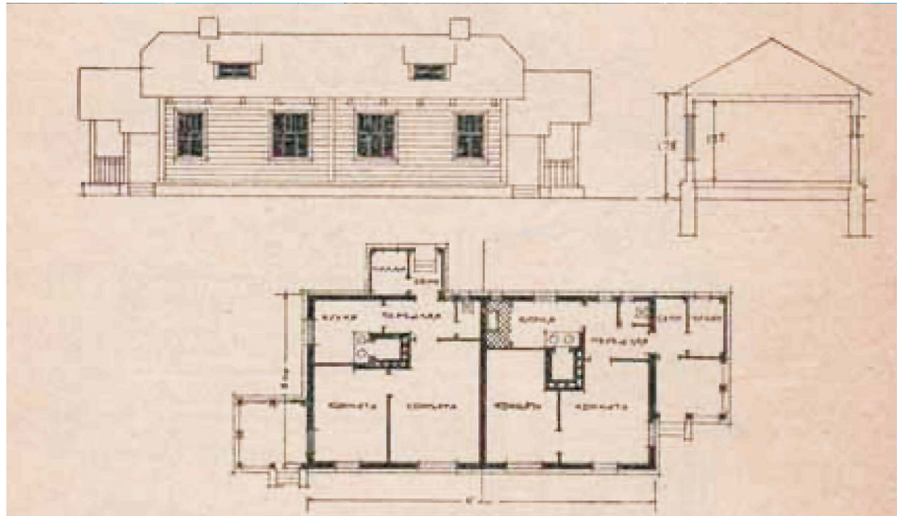
Проект двухквартирного дома для малосемейного рабочего
