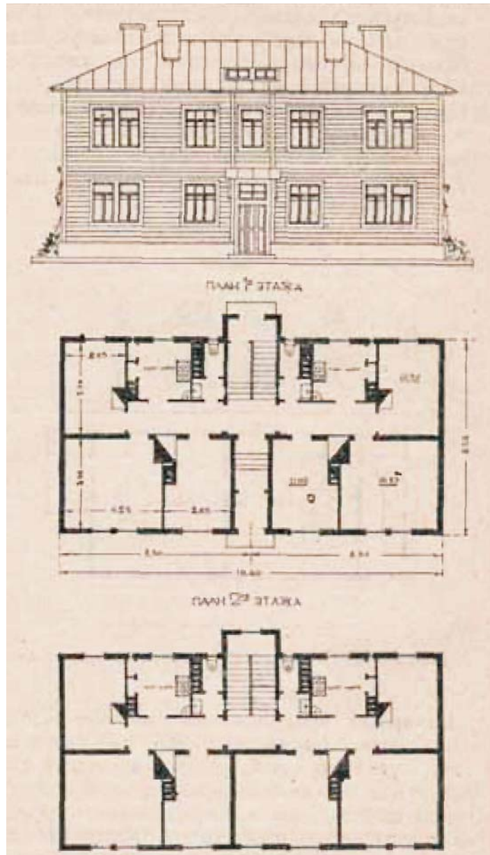
Мосгубжилсоюз. Проект деревянного четырехквартирного дома
