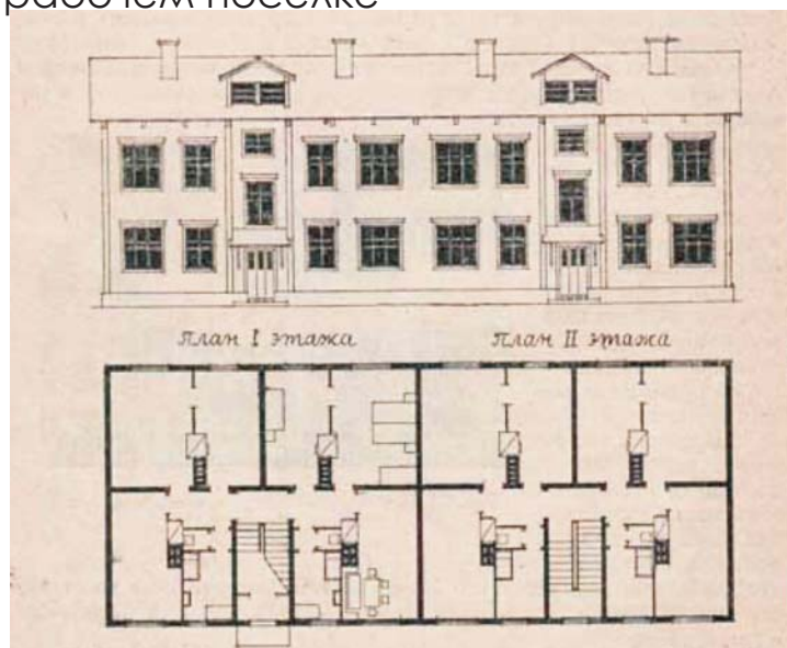
Проект восьмиквартирного дома на Дедовской фабрике Красно-Пресненского треста, тип Б
