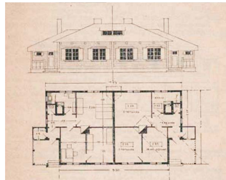
Проект двухквартирного дома
